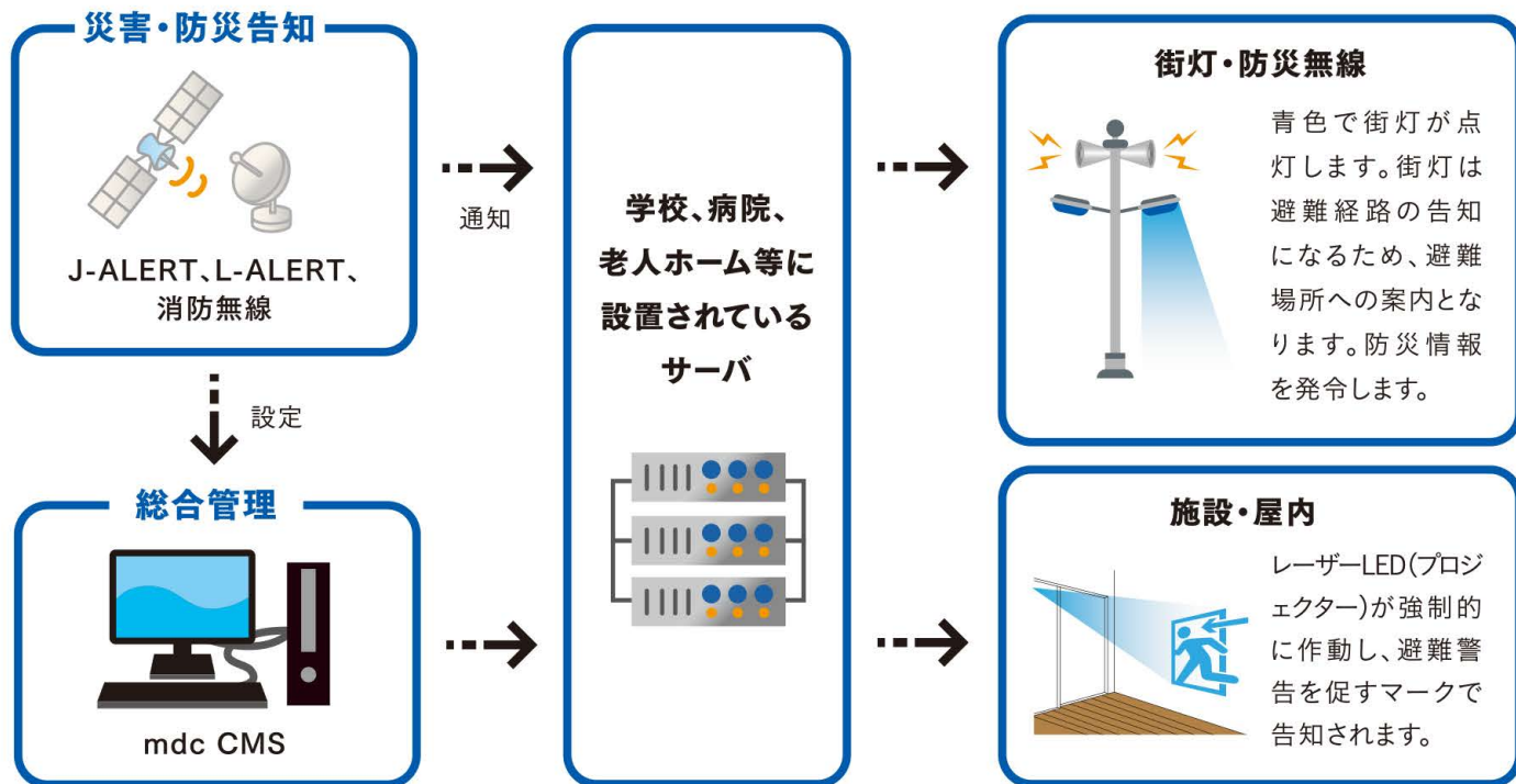
災害情報発令後の各設備の動作イメージ
